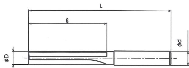
φD公差
