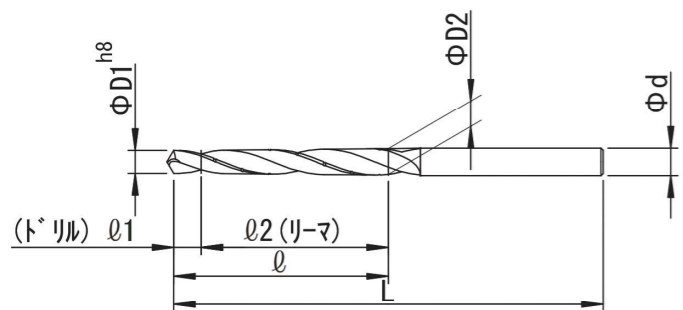
1/50テーパー 右刃右ネジレ 刃数2 SKH56 1/50Taper Helix Angle-Right 2Flutes HSS-Co.
