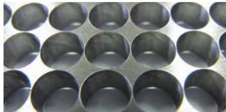
SUS 304 湿式穿孔 S=1280 F=51 V=24.1 f=0.039
