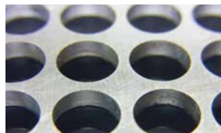
アルミ裏面 (CFRTP+アルミ同時穿孔) S=2660\text{rpm} F=37\text{mm}
